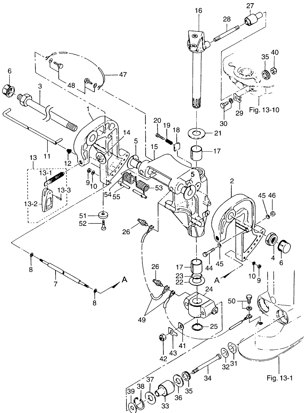
ブラケット Fig. 17 BRACKET
