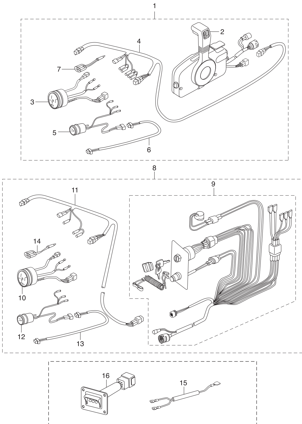
リギングキット Fig. 35 RIGGING KIT
