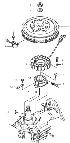
マグネト Fig. 9 MAGNETO
