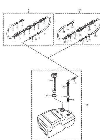
セパレートフュエルタンク Fig. 27 SEPARATE FUEL TANK
