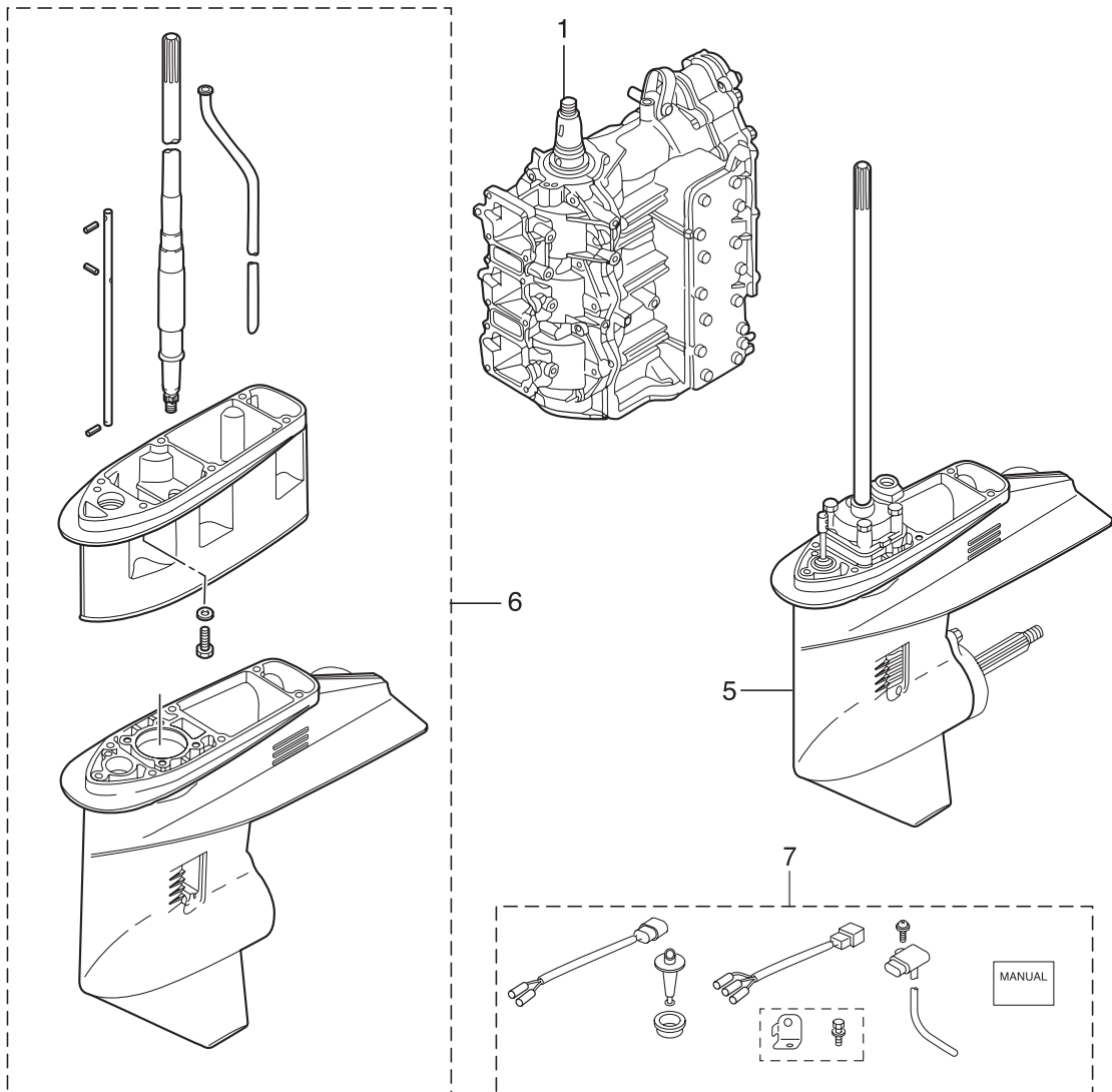
アッセンブリキット Fig. 34 ASSEMBLY・KIT
