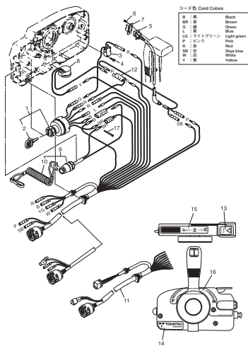
オプションパーツ (2) (P タイプ) Fig. 32 OPTIONAL PARTS (2)
