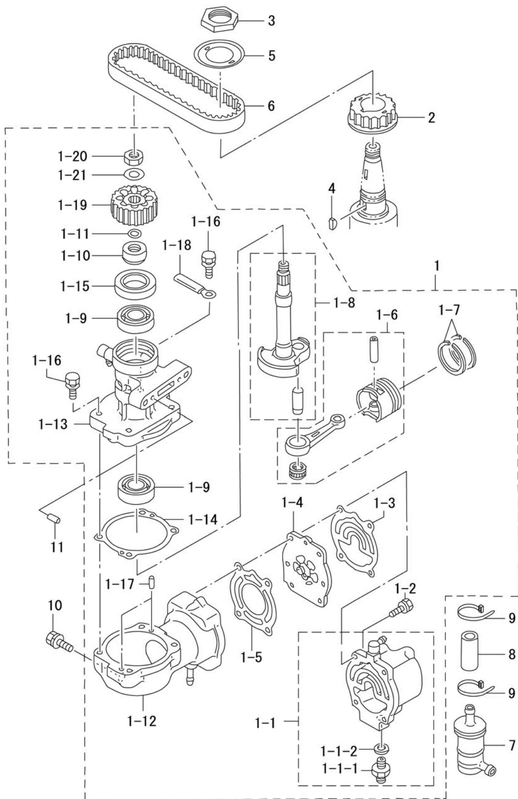
Fig.11 エアコンプレッサ AIR COMPRESSOR
