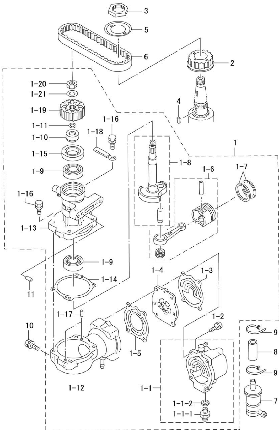
Fig.13 エアコンプレッサ AIR COMPRESSOR
