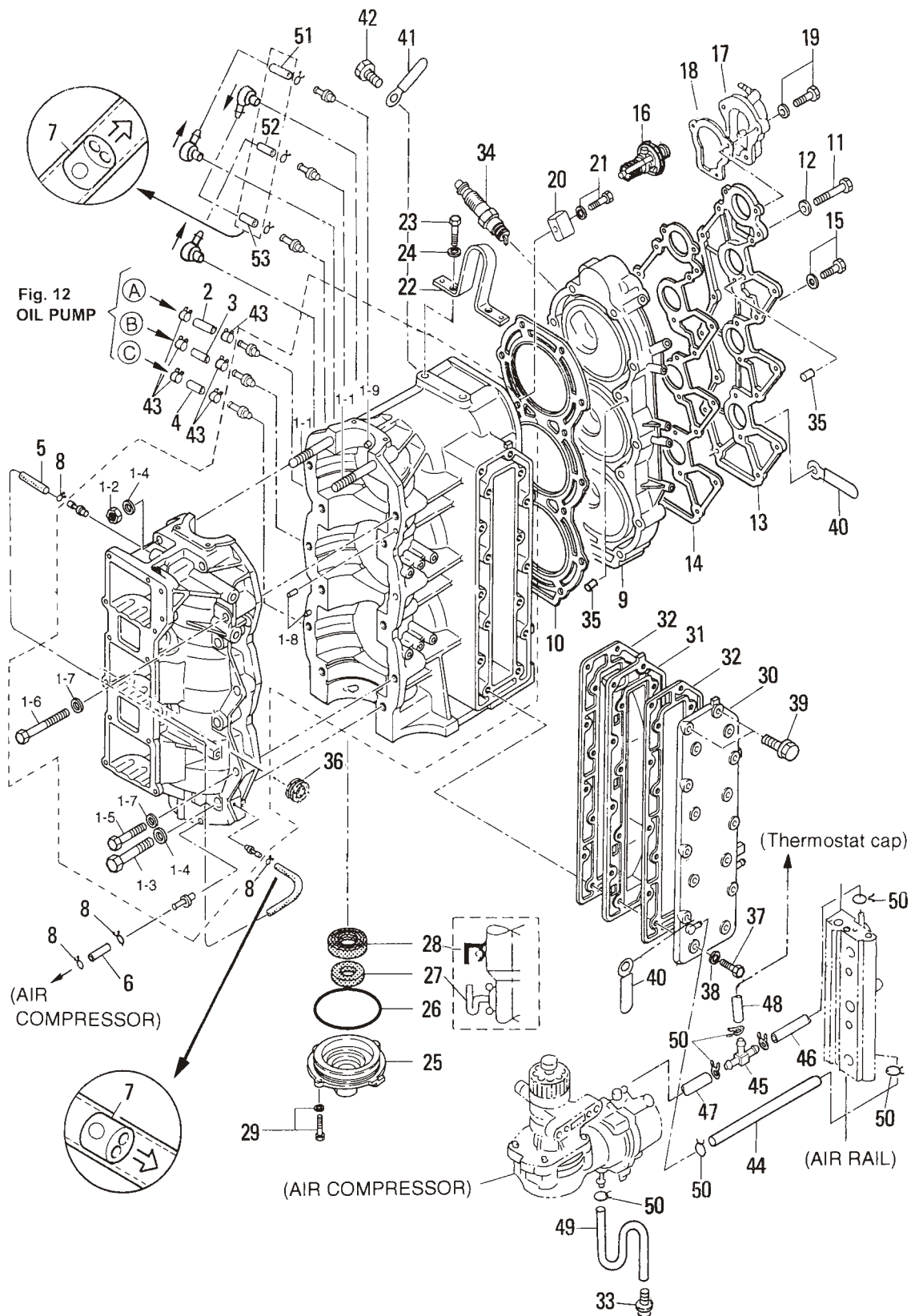
シリンダ・クランクケース CYLINDER・CRANK CASE Fig.1
