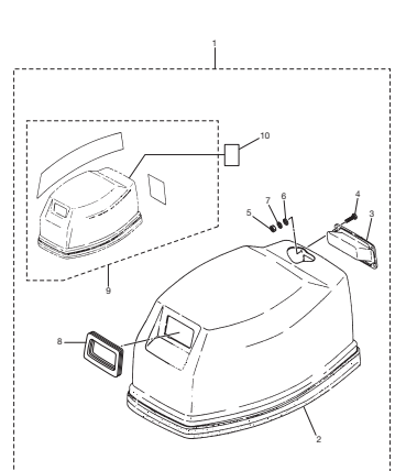
Fig.15 TOP COWL トップカウル
