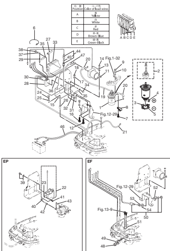
Fig. 7 ELECTRIC PARTS エレクトリックパーツ
