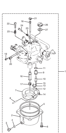
Fig. 4 CARBURETOR キャブレタ
