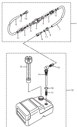
Fig.16 FUEL TANK フエルトンク
