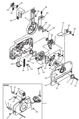
Fig.18 COMPONENT PARTS OF REMOTE CONTROL リモコンボックス構成部品
