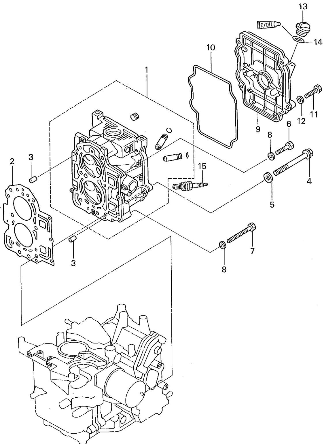
シリンダヘッド Fig. 1 CYLINDER HEAD
