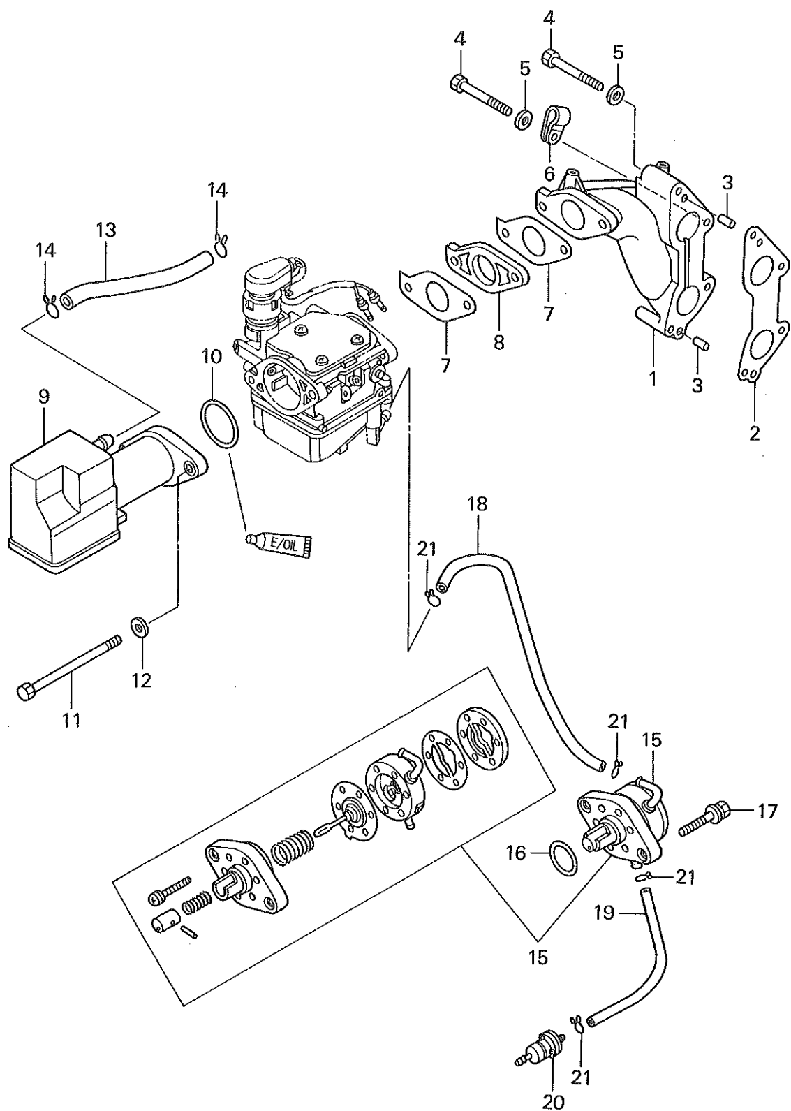
Fig. 4 インレットマニホールド & フュエルポンプ INLET MANIFOLD & FUEL PUMP
