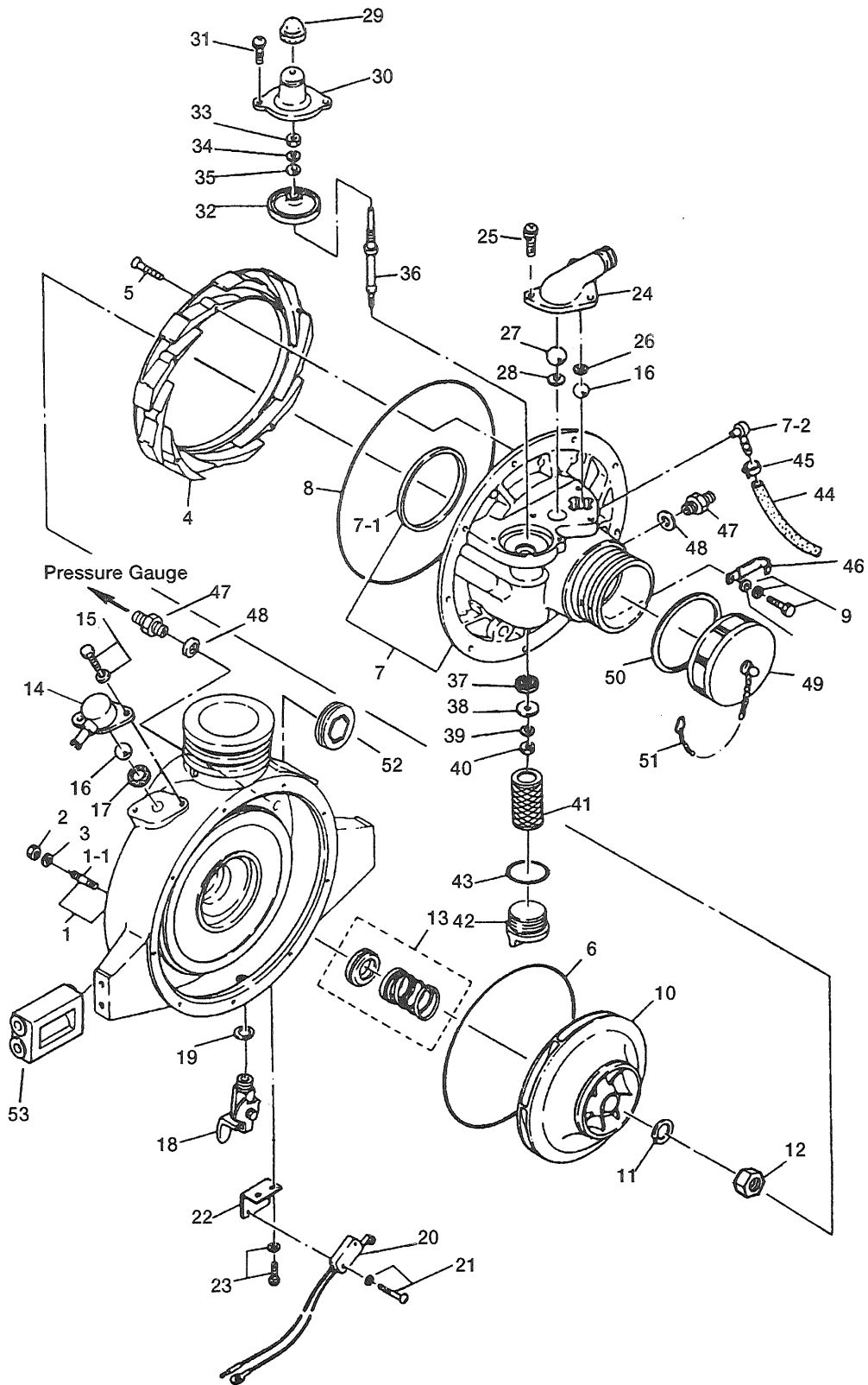
ポンプケース Fig. 11 PUMP CASE
