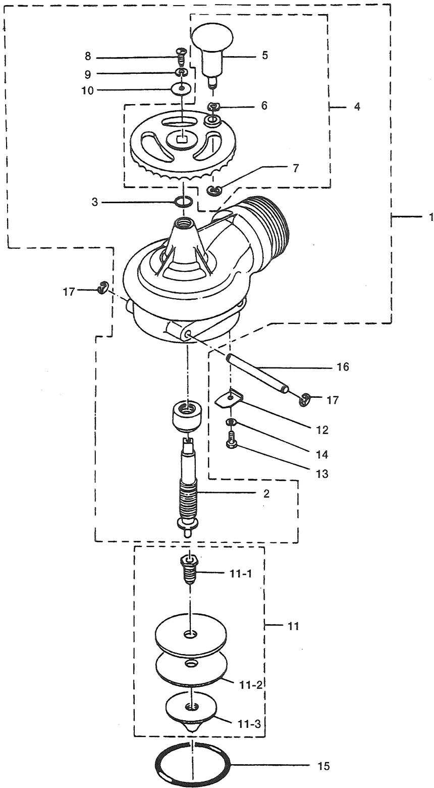
ディスチャージバルブチャンバー Fig. 13 DISCHARGE VALVE CHAMBER
