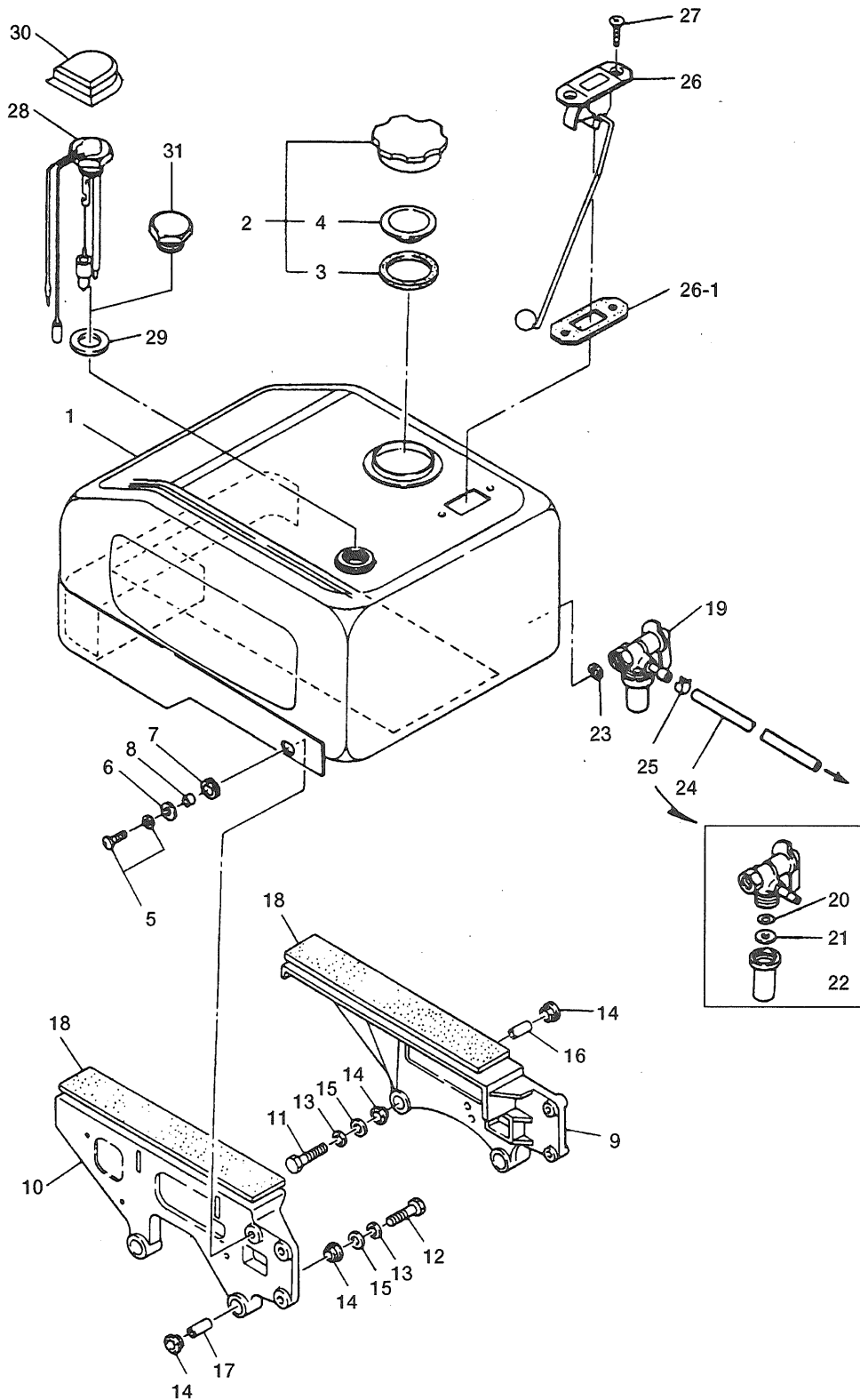
フュエルタンク Fig. 18 FUEL TANK
