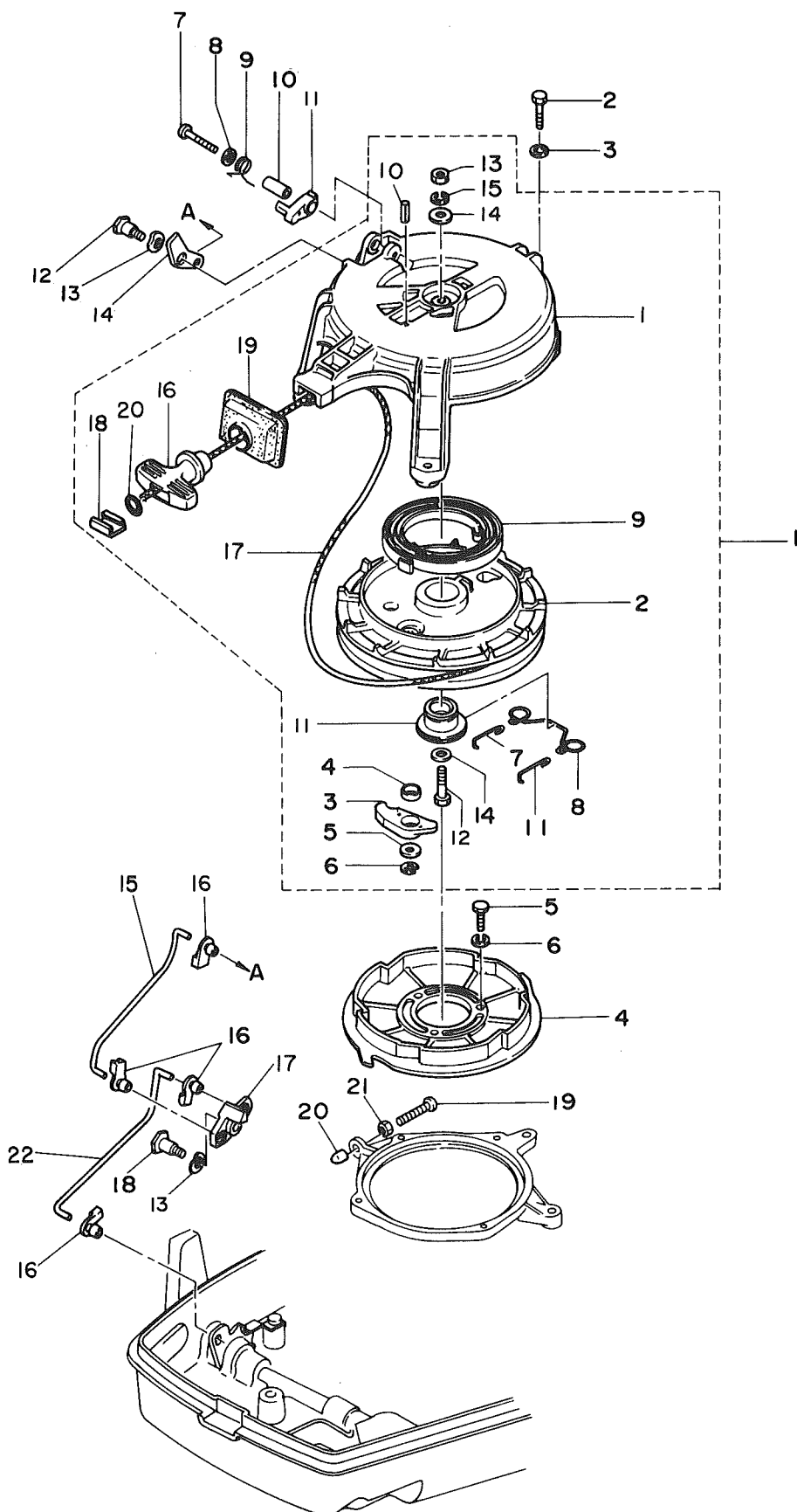
Fig.7-A リコイルスタータ・スタータロック RECOIL STARTER・STARTER LOCK
