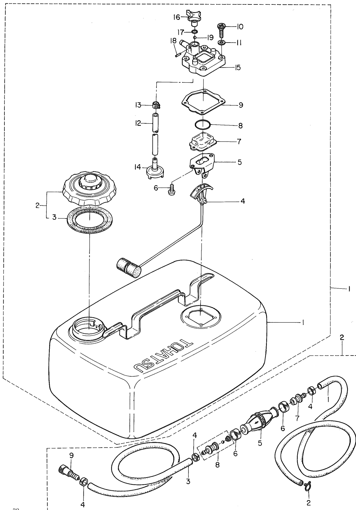
フュエルタンク Fig. 13-A FUEL TANK
