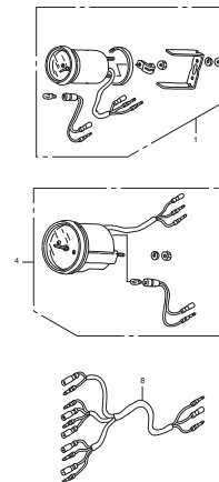
FOP-5-1 METER
