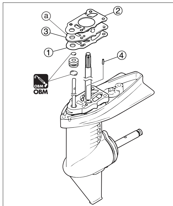
a突起 ①② 再使用不可
