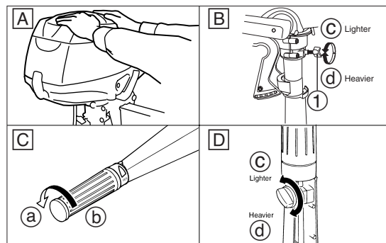
①ステアリングアジャストスクリュー Ⓒ軽く Ⓓ重く
