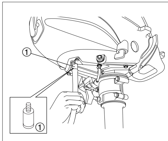
①フラッシングアタッチメント（オプション）
