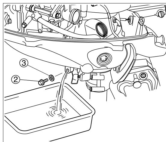
③ワッシャ 再使用不可
