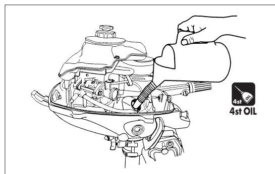
①オイルフィルターキャップ
