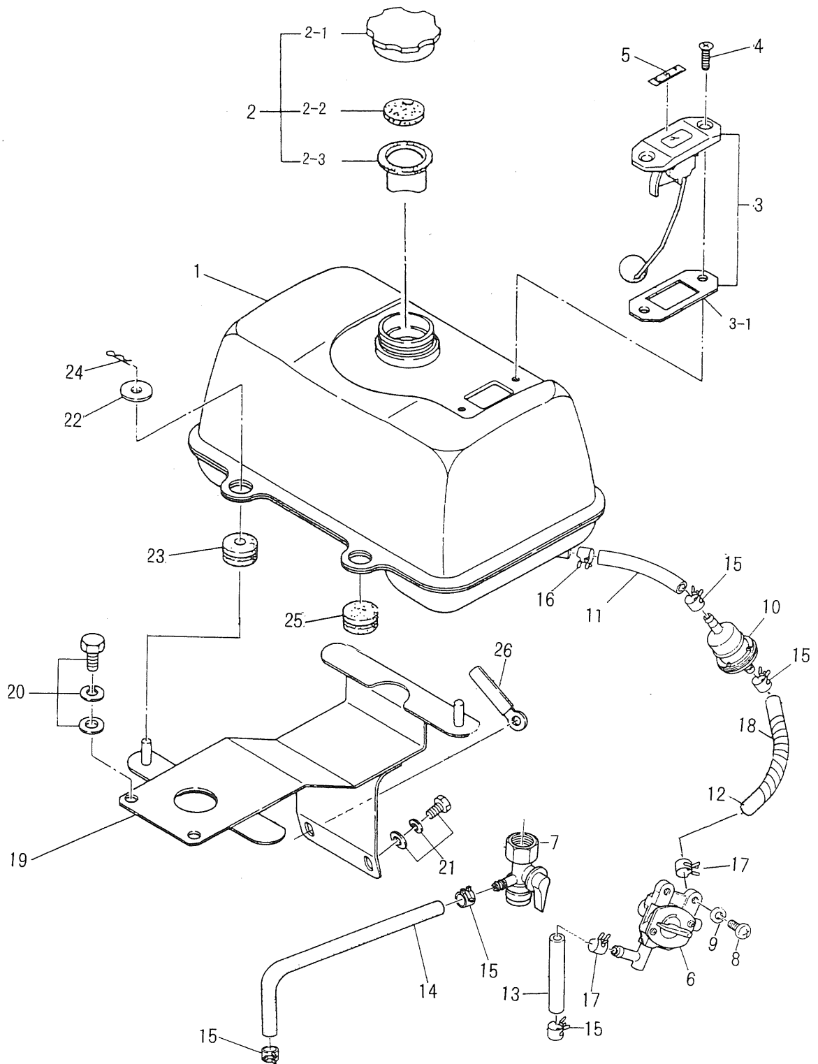
Fig. 14 フュエルタンク FUEL TANK
