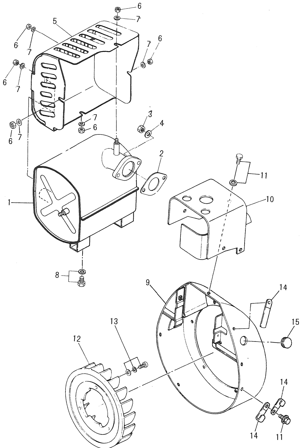
マフラ・ファンケース Fig. 5 MUFFLER·FAN CASE
