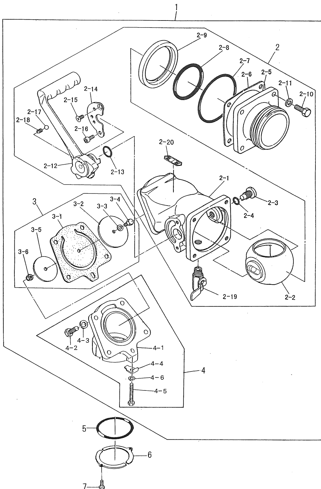
オフティバルブ(V20ES-R) Fig. 13 DISCHARGE VALVE CHAMBER
