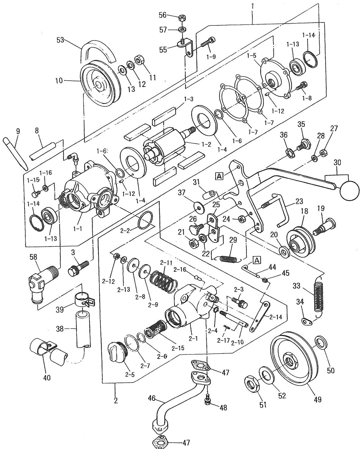
ハキウムポンプ (V20ES-R) Fig. 12 VACUUM PUMP
