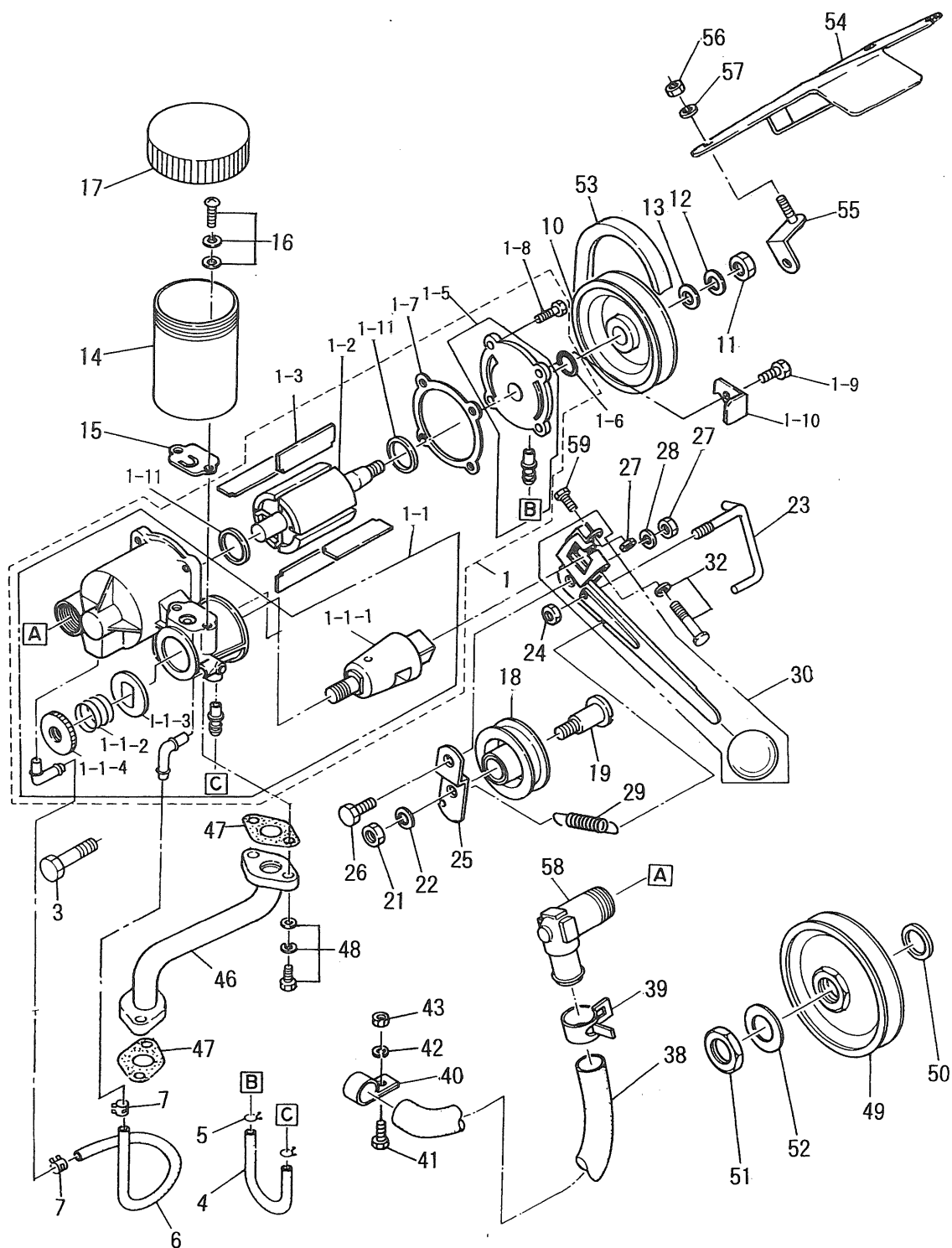
バキュームポンプ (V20JE) Fig. 12B VACUUM PUMP
