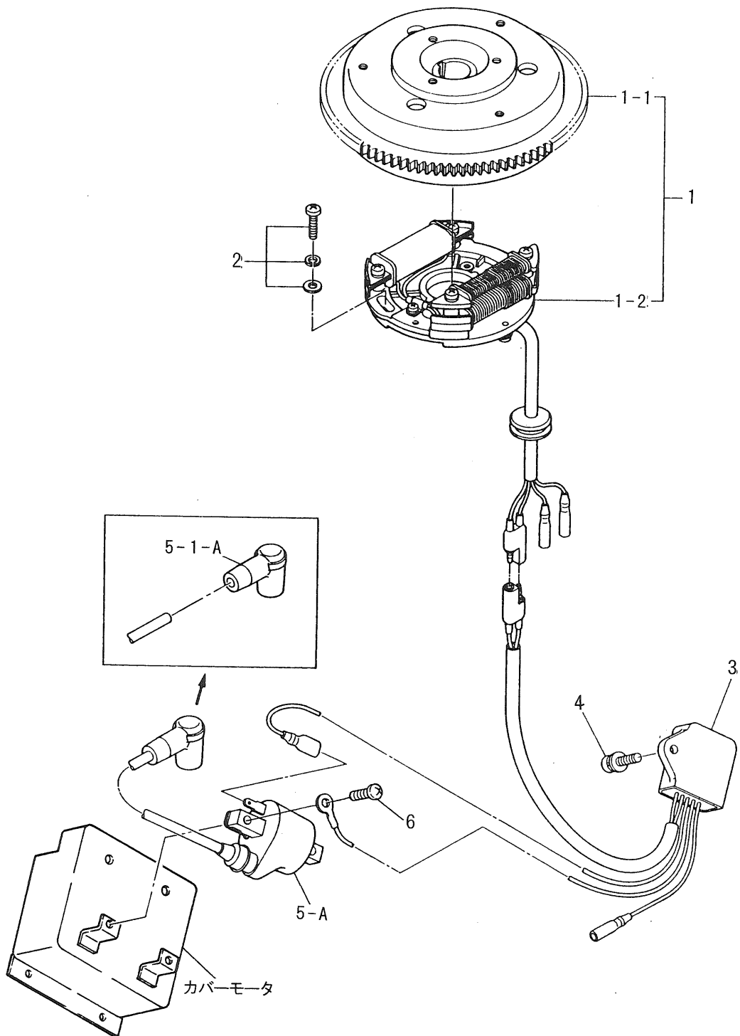
マグネト (V20ES-R) Fig. 6-A MAGNETO
